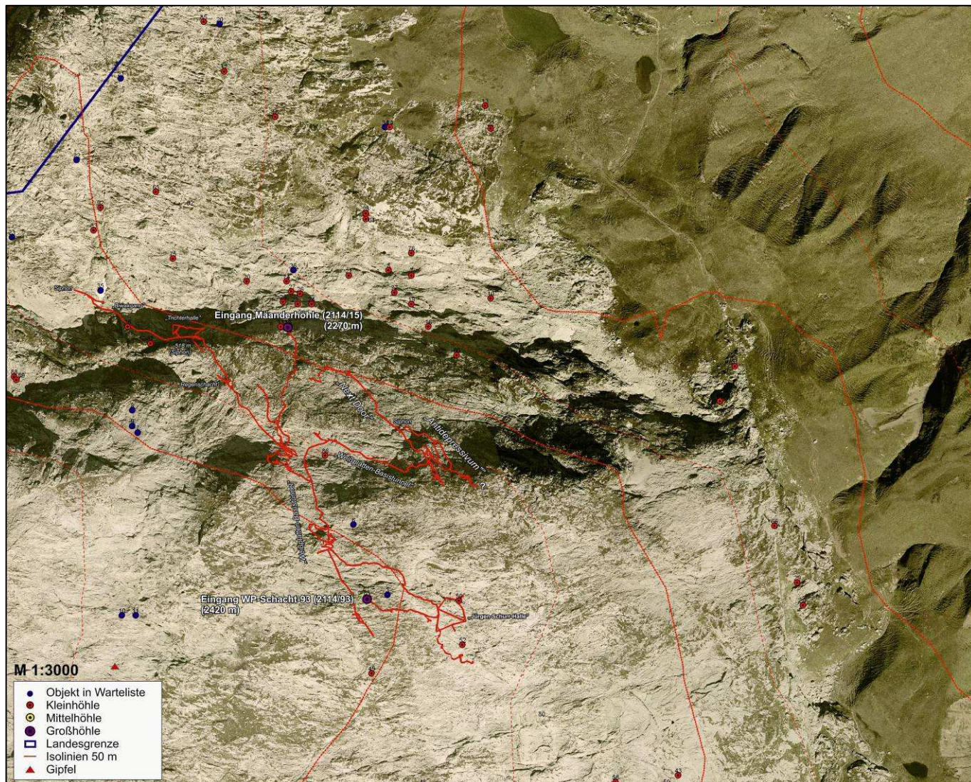
Übersicht über das Weißplattenhöhlensystem (Stand: September 2013)
